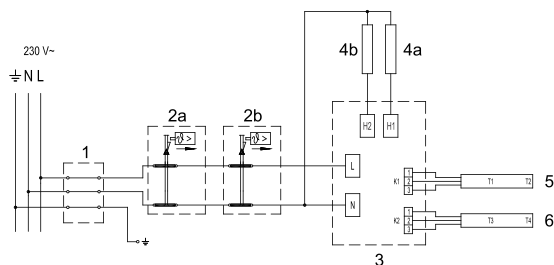
Sl. 6: Električna spojna shema
