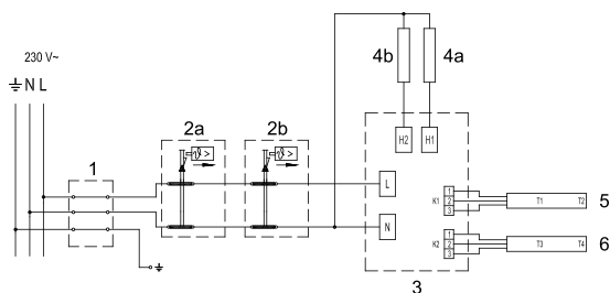
Sl. 6: Shema električne vezave
