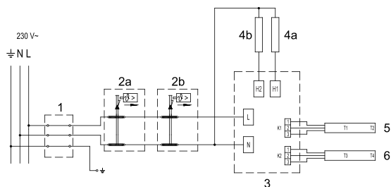
Sl. 6: Šema povezivanja električnih provodnika
