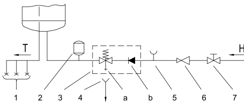
Abb. 3: Geschlossenes System (druckfestes System)
