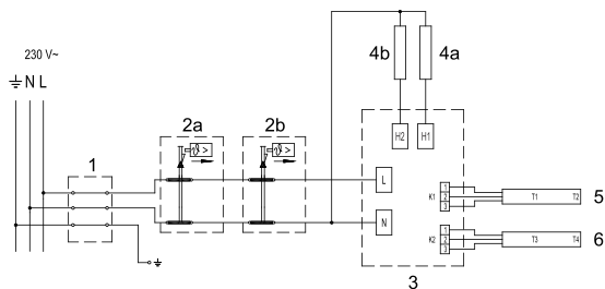
Abb. 6: Elektroschaltbild
